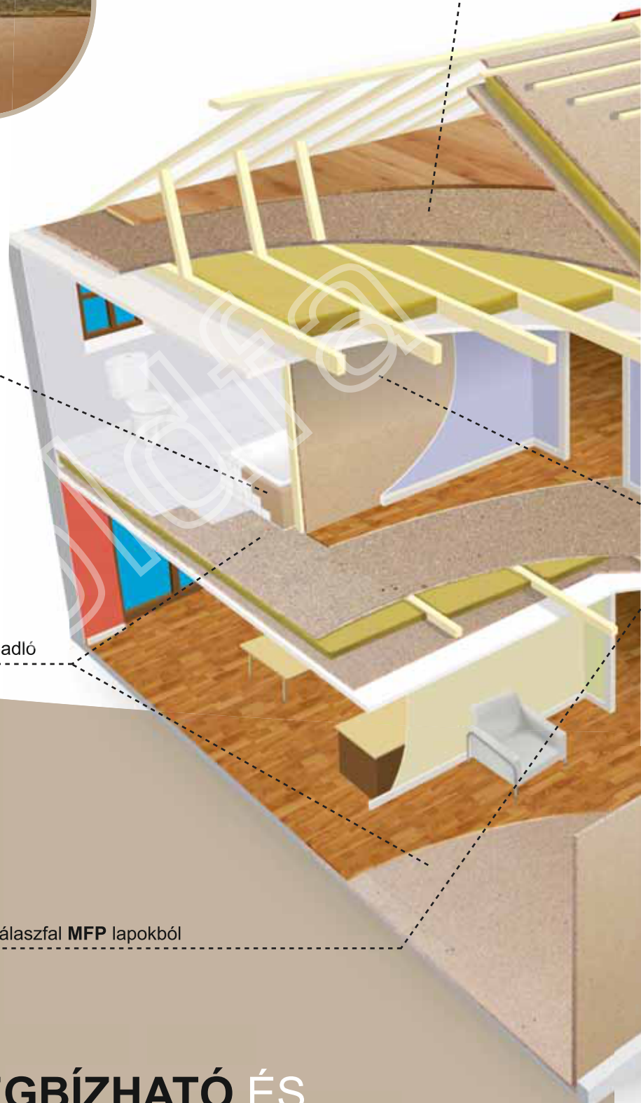
MFP lapokból készült szerkezeti elemek
